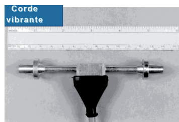
Corde vibrante du type TELEMAC C110 (IFSTTAR)
